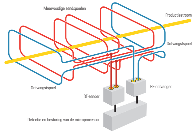
APEX meerspoelige detectorconstructie
